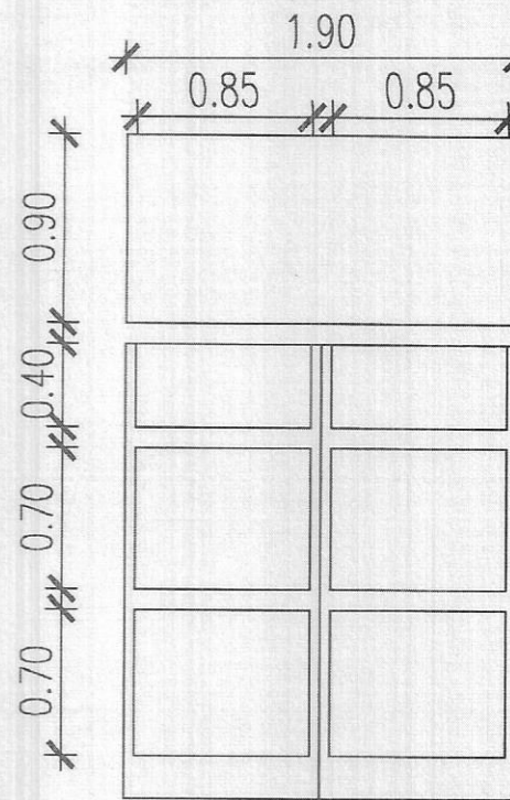
Puerta Sec. de 2 hojas vidrio repartido con Paño Fijo (Av. Belgr.)
