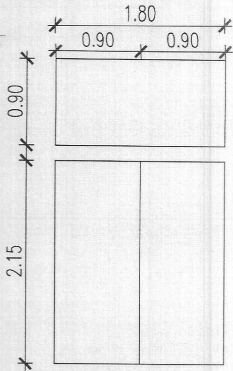
Puerta Prin. pivote de 2 hojas con Paño Fijo (Ochaba)
